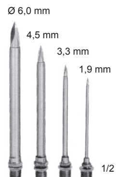
TROCATER UNIVERSAL COM 4 PONTAS BW-464
